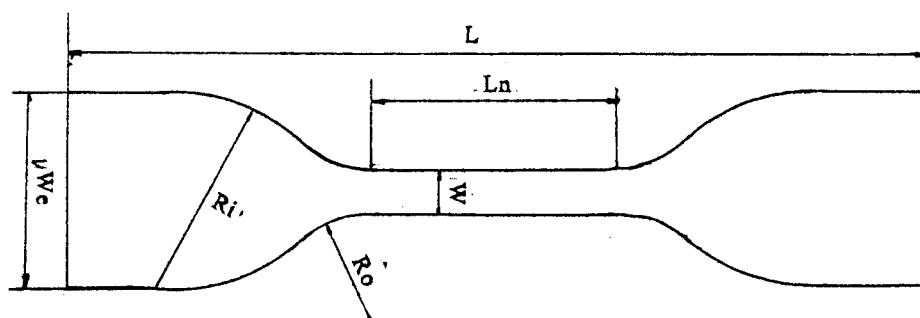
图1 哑铃型试样裁刀
